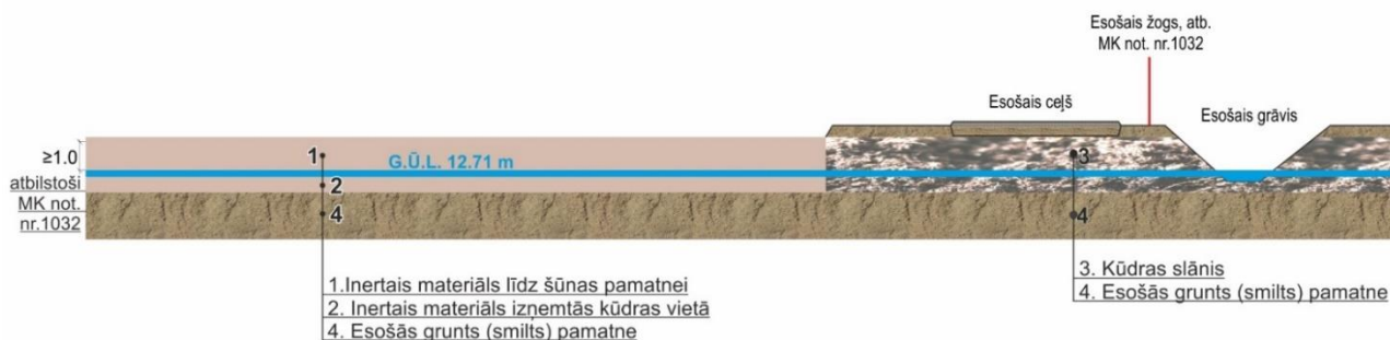
3.34. attēls. 1. būvniecības kārtā: griezum A-A
