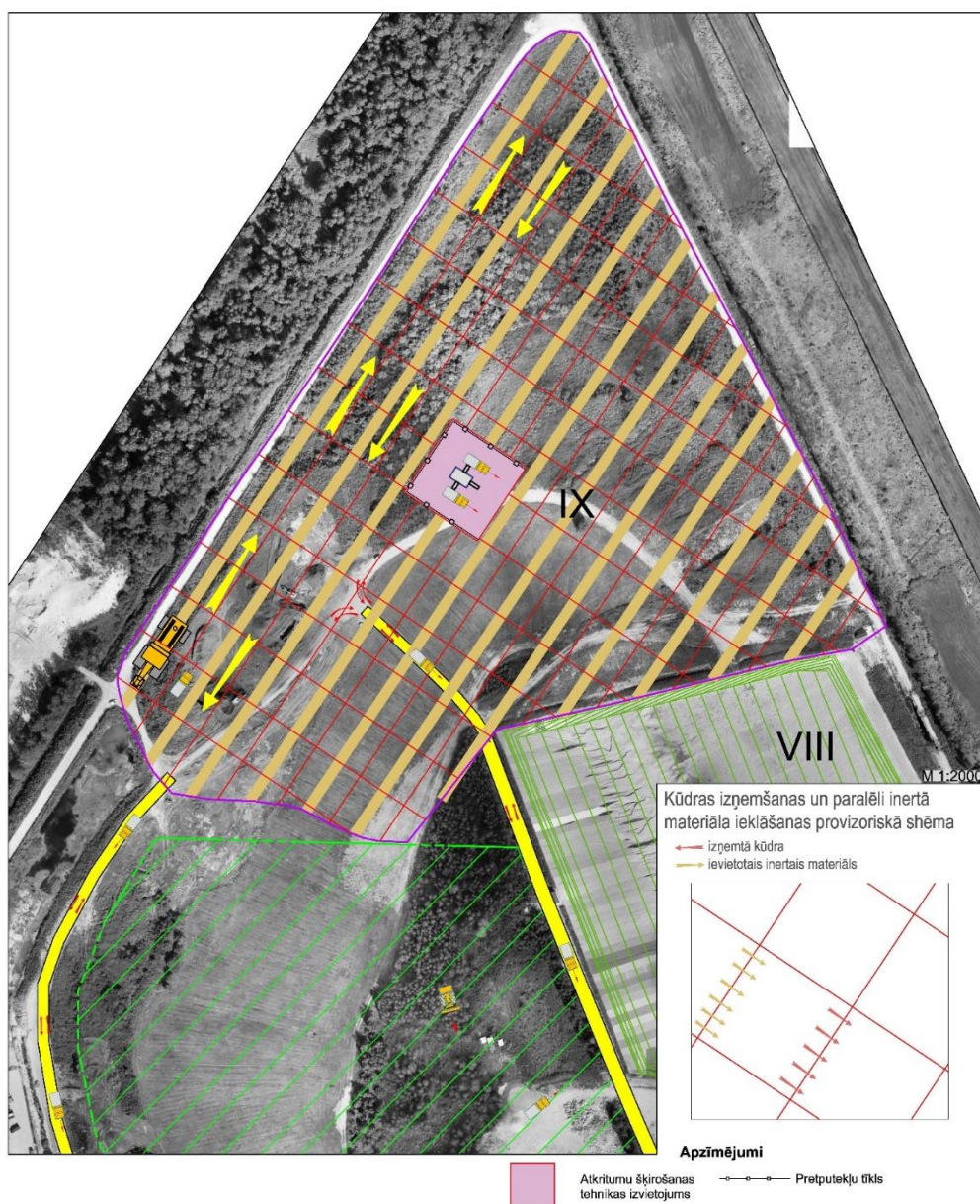
3.32. attēls. Būvdarbu organizācija 1. būvniecības darbu kārtā
