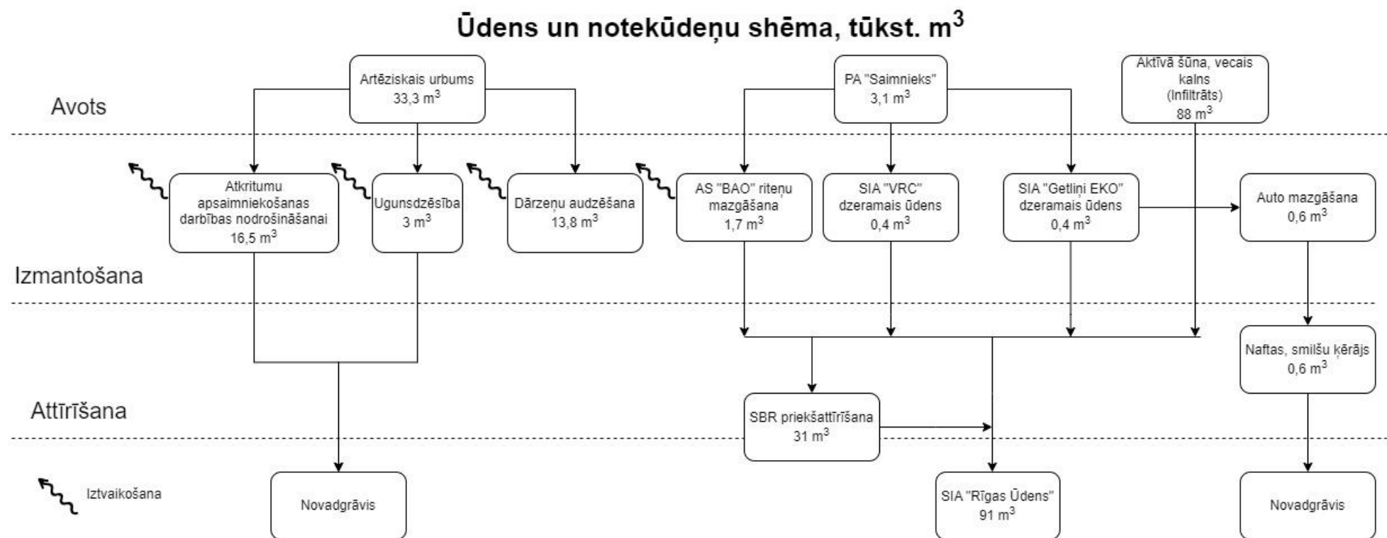
3.10. attēls. Sadzīves atkritumu poligona "Getliņi" ūdens resursu izmantošanas un notekūdeņu apsaimniekošanas sistēmas shēma
