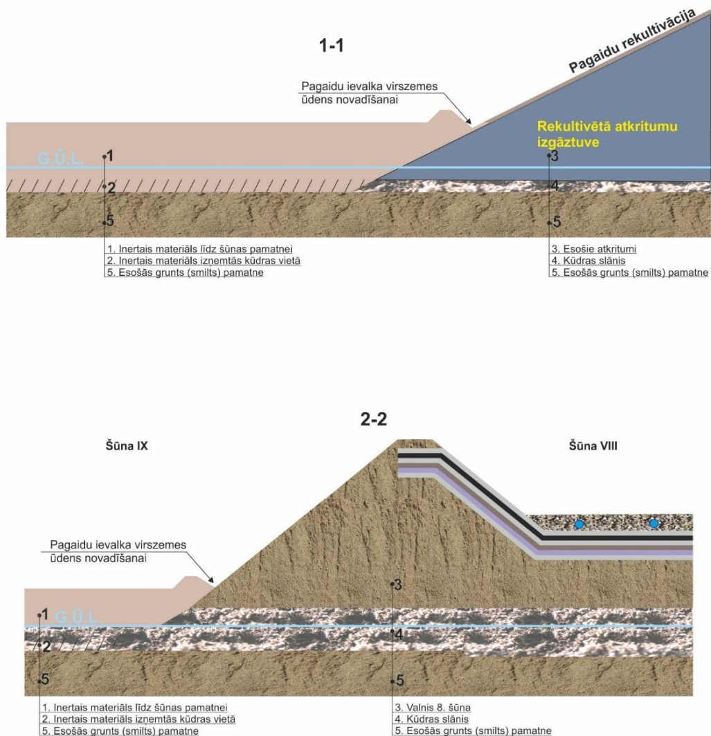
3.31. attēls. Būvniecības darbu 1. kārtā: rekultivācijas pārklājošā slāņa izņemšana, atkritumu izņemšana un inertās kārtas ievietošana. 1-1 griezum un 2-2 griezum
