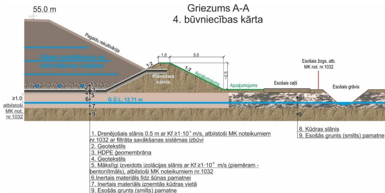
3.46. attēls. 4. būvniecības kārtā: griezums A-A
