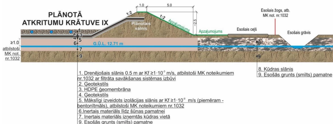
3.38. attēls. 2. būvniecības kārtā: griezum A-A
