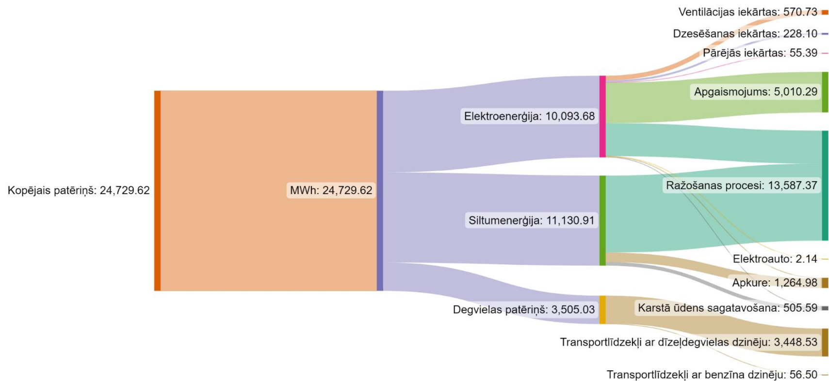
3.17. attēls. Enerģijas plūsmas diagramma (balance) (avots: SIA "LBRA" Inspekcija "SIA "Getliņi EKO" lielā elektroenerģijas patērētāja energoaudita pārskats", 2023. g.)
