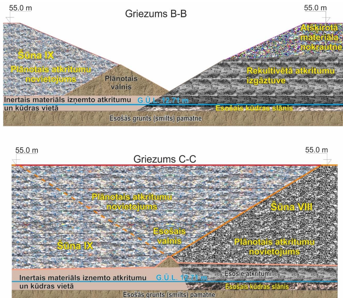
3.43. attēls. Griezums B-B un griezumā C-C
