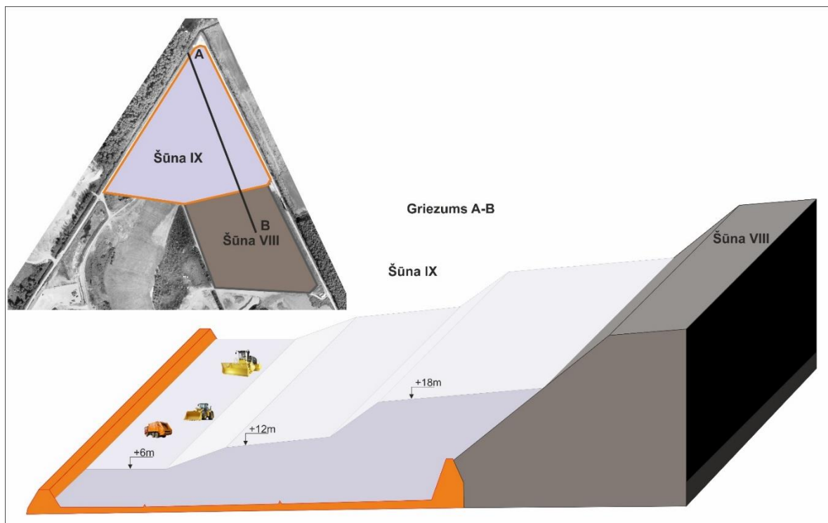
3.41. attēls. Šūnu aizpildīšanas (ekspluatācijas) tehnoloģiskā shēma
