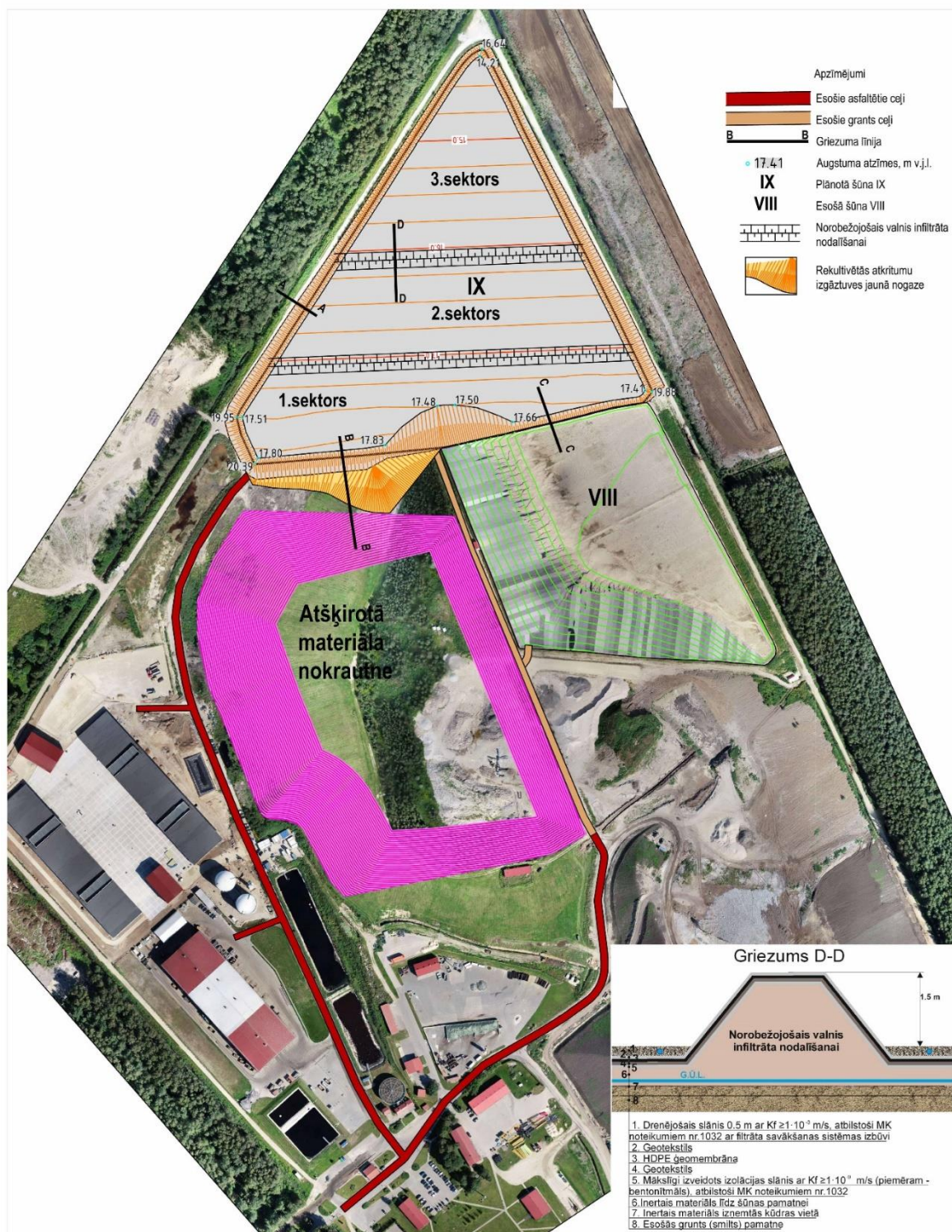
3.35. attēls. Šūnas Nr. IX izbūve poligona teritorijā, D-D griezumā
