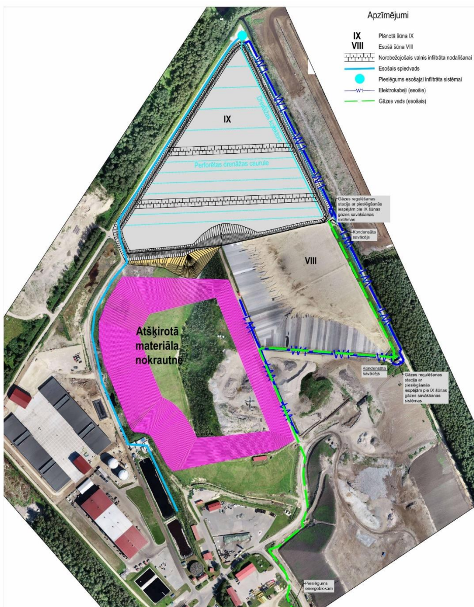
3.44. attēls. Pieslēgums pie esošajiem inženiertīkliem
