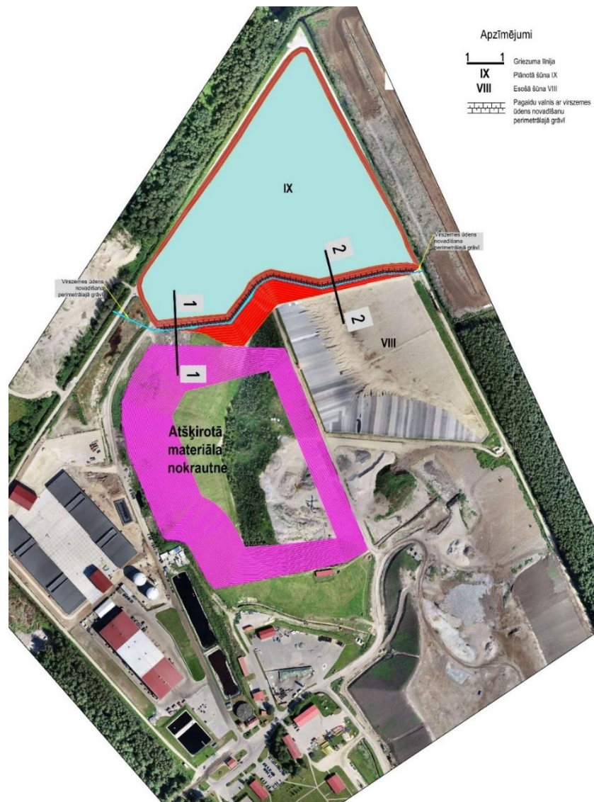
3.30. attēls. Būvniecības darbu 1. kārtā: rekultivācijas pārklājošā slāņa izņemšana, atkritumu izņemšana un inertās kārtas ievietošana, 1-1 griezuma un 2-2 griezuma izvietojums
