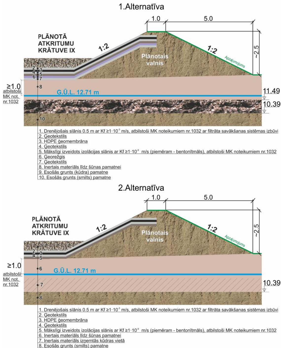
4.3. attēls. 1. alternatīvas un 2. alternatīvas atkritumu apglabāšanas šūnas Nr. IX uzbūve (shematisks zīmējums)
