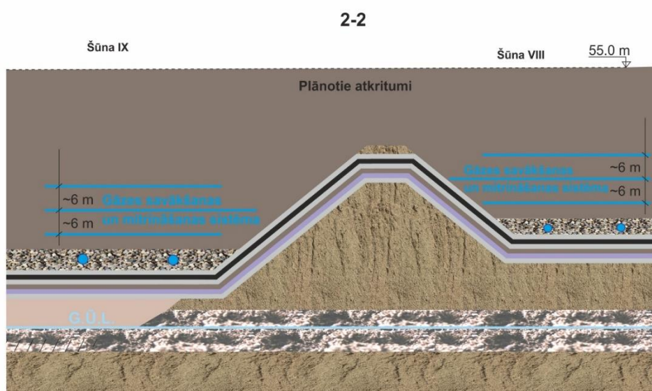
3.40. attēls. Būvniecības darbu 3. kārtā: Atkritumu aizpildīšana un gāzes savākšanas sistēmas izbūve šūnā Nr. IX un šūnā Nr. VIII. 1-1 griezum un 2-2 griezum
