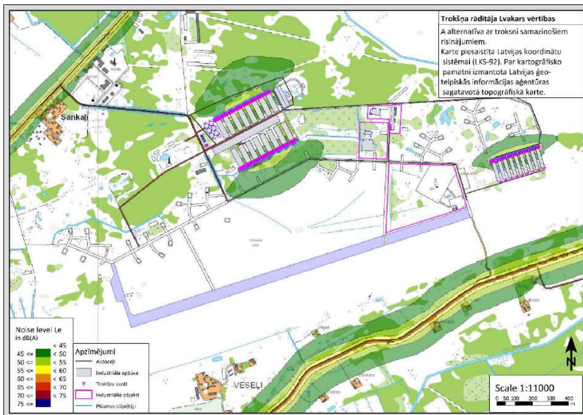
16. attēls. Radītā trokšņa radītāja Lnakars vērtības, A alternatīva ar troksni samazinošiem risinājumiem.
