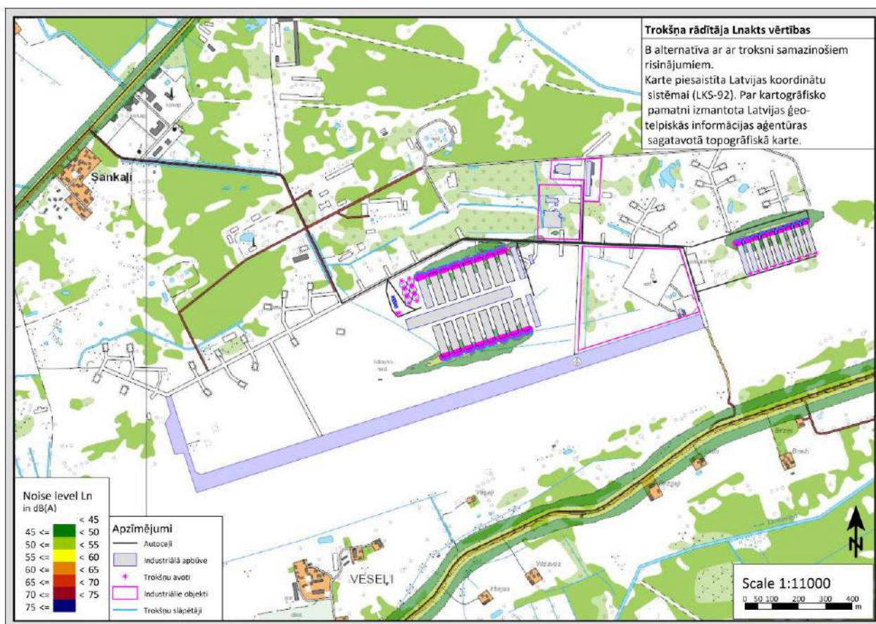
20. attēls. Radītā trokšņa rādītāja Lnakts vērtības, B alternatīva ar troksni samazinošiem risinājumiem.
