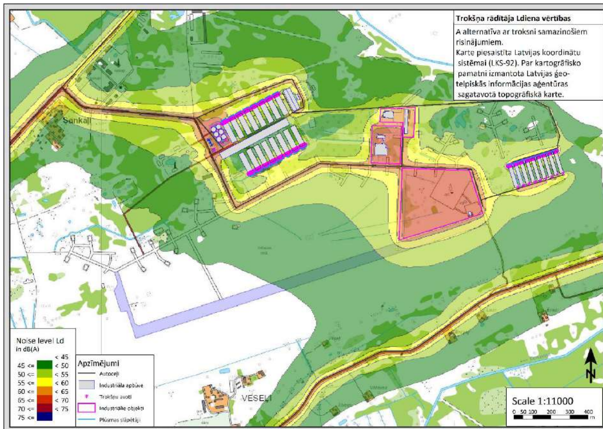
15. attēls. Radītā trokšņa radītāja Ldienas vērtības, A alternatīva ar troksni samazinošiem risinājumiem.
