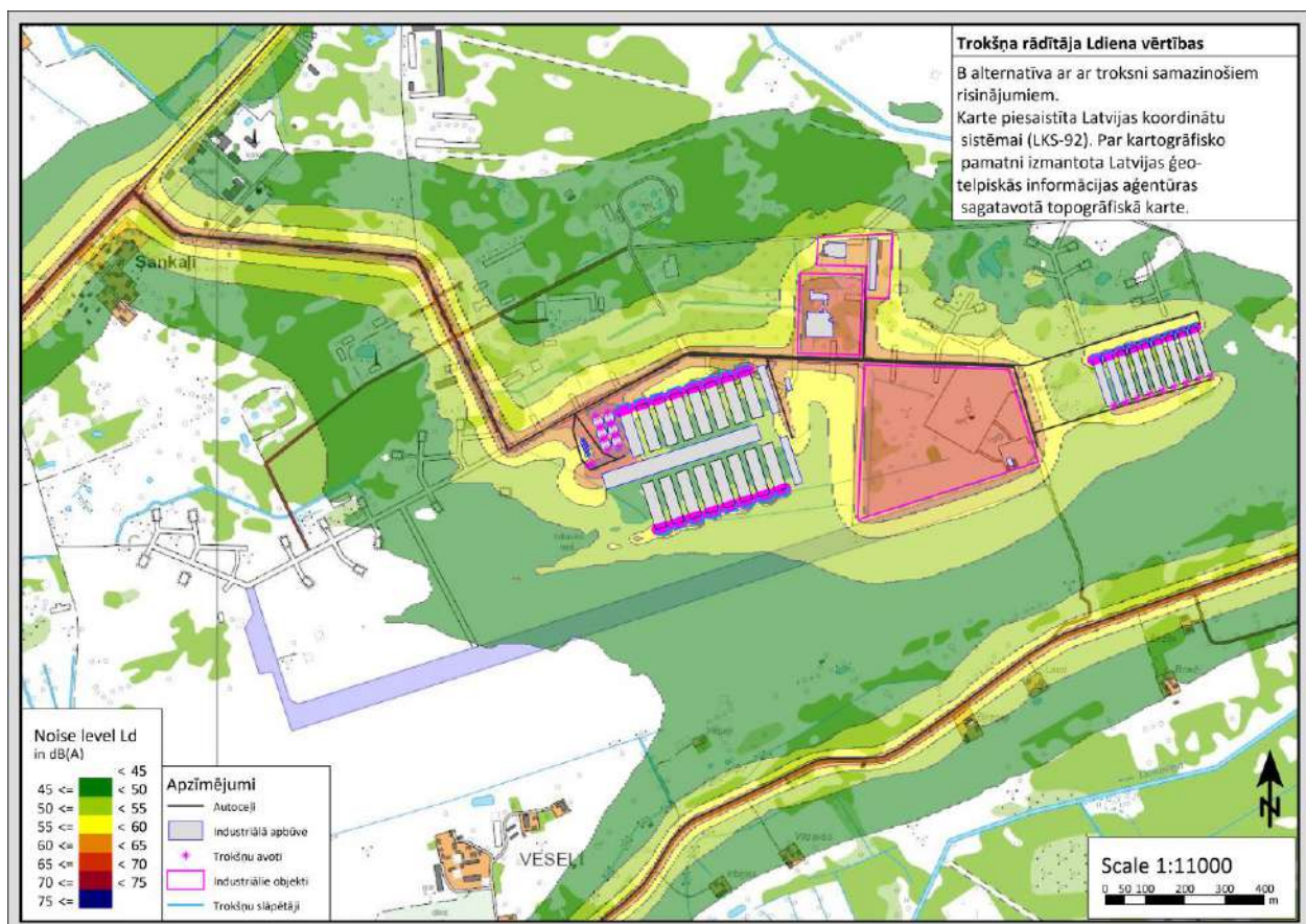
18. attēls. Radītā trokšņa rādītāja Ld akts vērtības, B alternatīva ar troksni samazinošiem risinājumiem.
