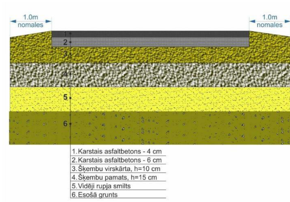
3.30. attēls. Jaunā ceļa principiālais šķēršporfils
