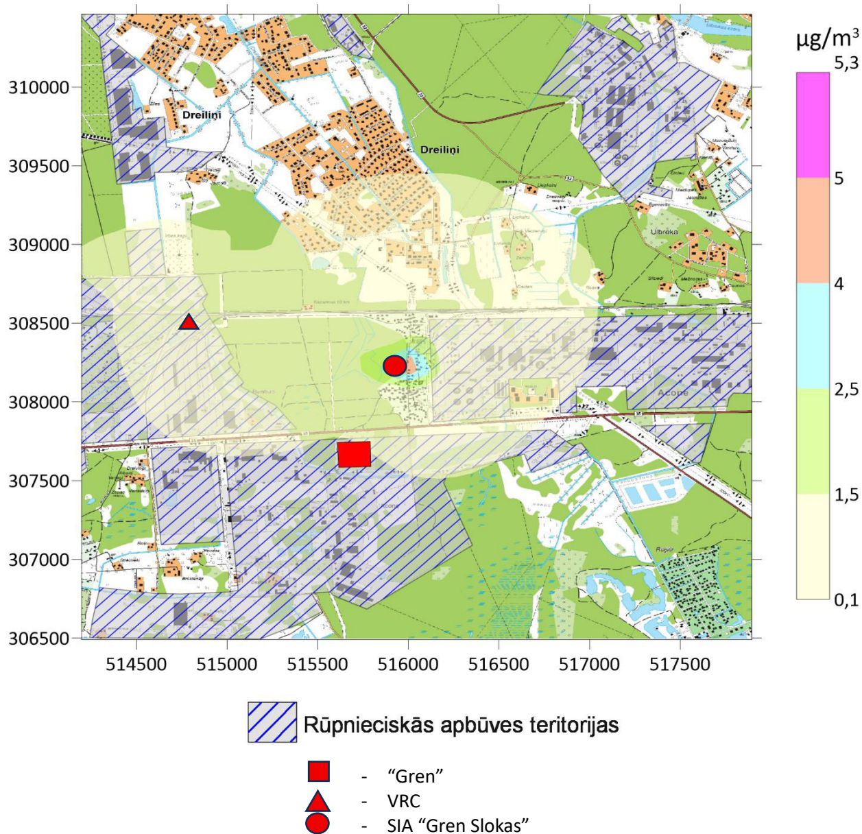
3.18. attēls. Summārā PM_{10} emisiju dispersija "Gren", VRC un SIA "Gren Slokas" paredzētās darbības gadījumā gada intervālā ieskaitot fona koncentrācijas
