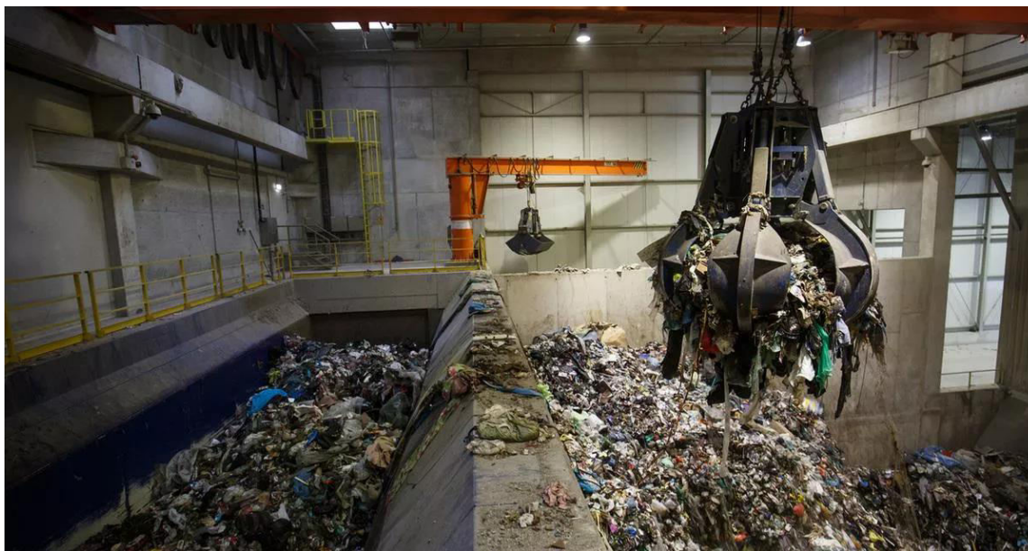
3.8. attēls. Bunkurs un greifera kauss (avots: Spectra, 2023 5 )
