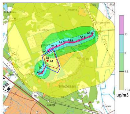
PM 10 gada vidējo koncentrāciju novērtējums
