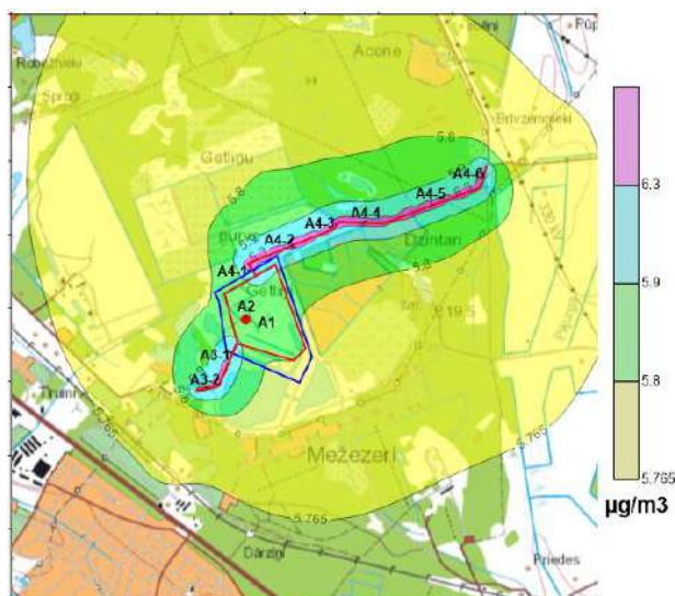
PM 2.5 gada vidējo koncentrāciju novērtējums
