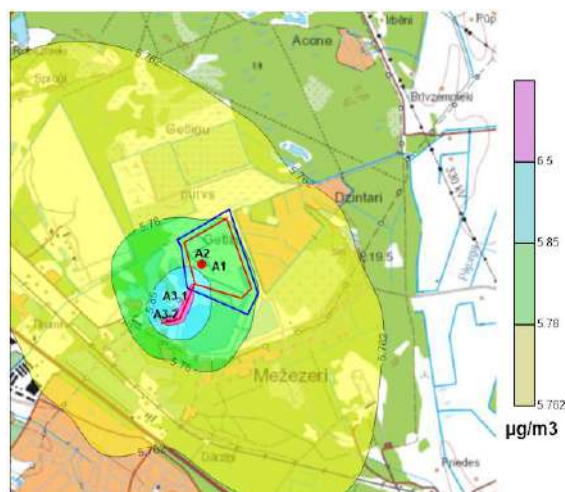
PM 2.5 gada vidējo koncentrāciju novērtējums
