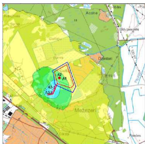
PM 10 diennakts 35.augstākās koncentrācijas novērtējums
