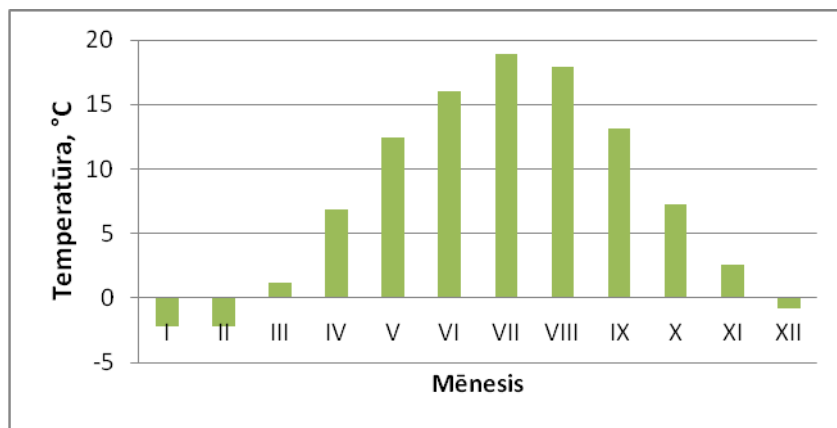
2.8. attēls. Vidējā gaisa temperatūra (ilggadīgie novērojumi) (meteoroloģiskā stacija "Rīga")
