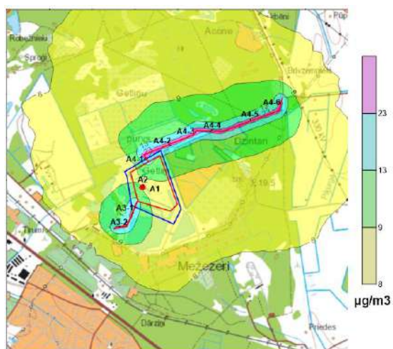
PM 10 diennakts 35.augstākās koncentrācijas novērtējums
