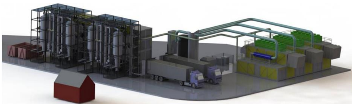
Attēls 12. Attēls. NAIK gazifikācijas iekārta ar izejmateriāla iekraušanu tieši no autotransporta
