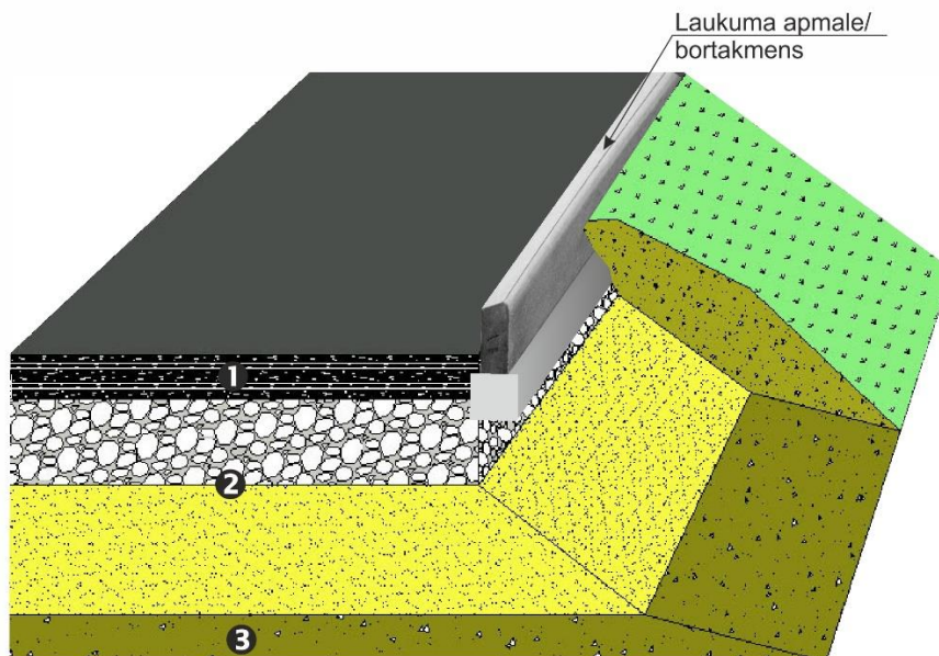
Laukuma konstrukcija
