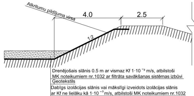
Griezums 1-1
