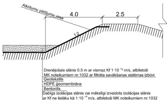
Griezums 2-2
