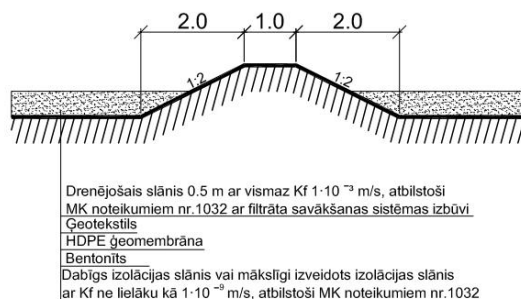
Griezums 3-3
