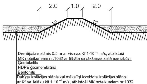
Griezums 3-3
