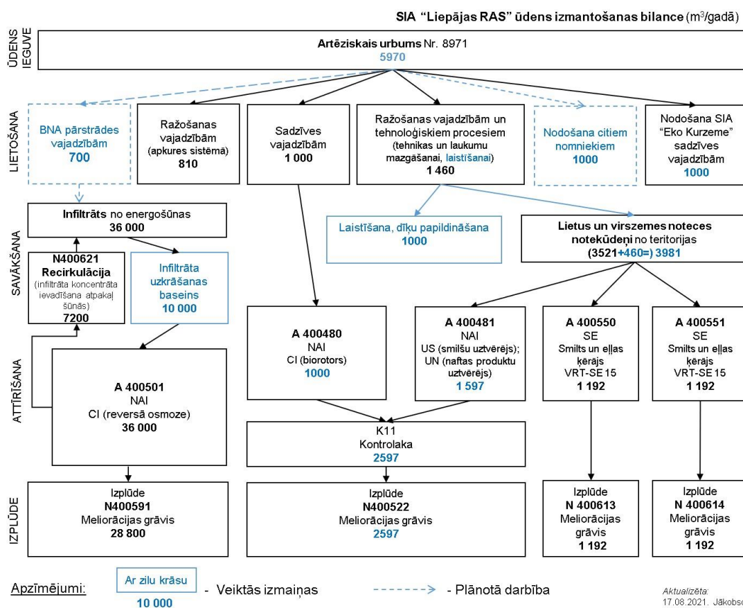
3.11. attēls. SIA “Liepājas RAS” plānotā ūdens izmantošanas balance (m 3 /gadā) (avots: SIA “Liepājas RAS”)
