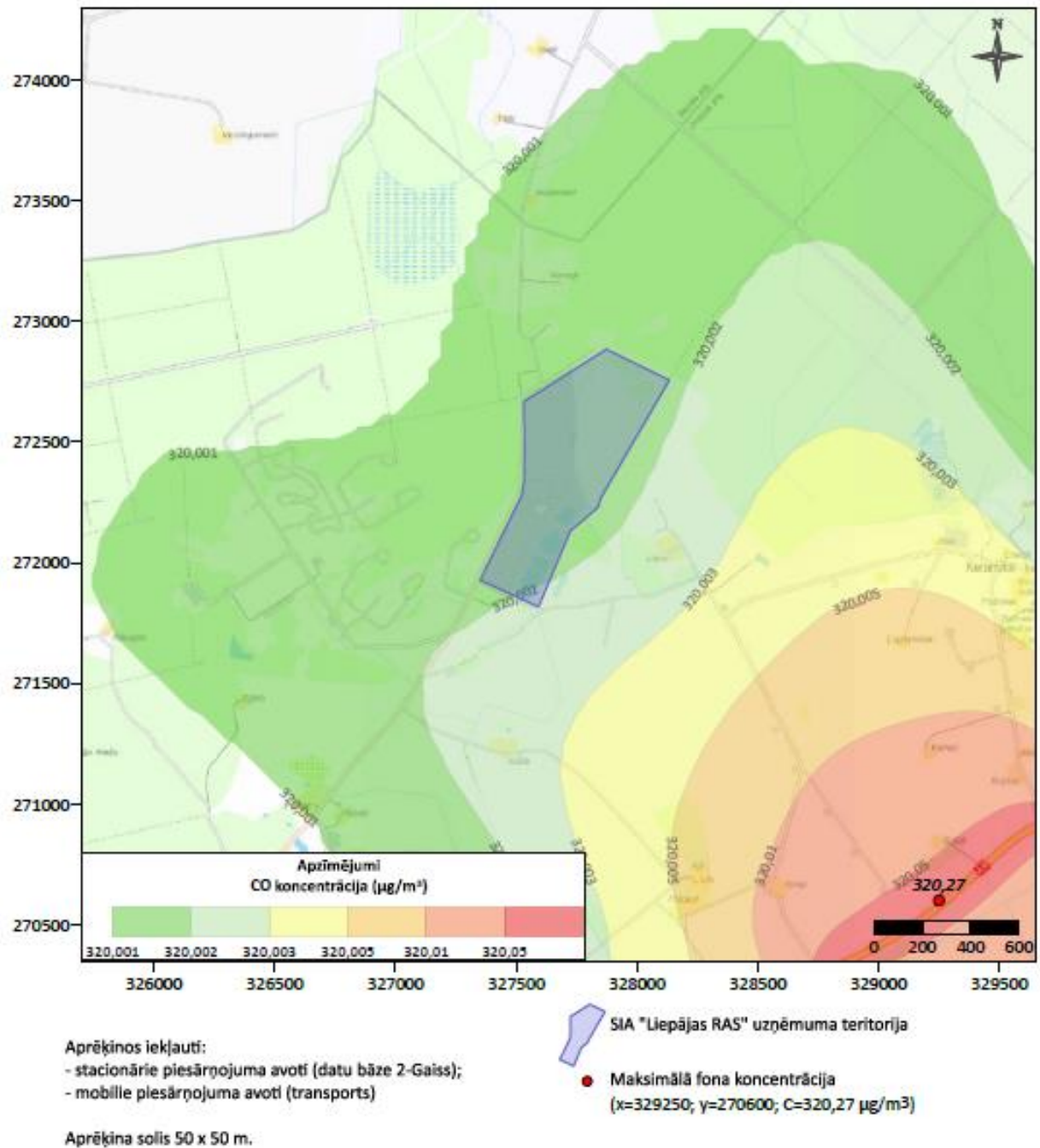
3.13. attēls. Oglekļa oksīda gada vidējo koncentrāciju novērtējums, fona piesārņojuma koncentrācija (avots: SIA "Ekosoft")
