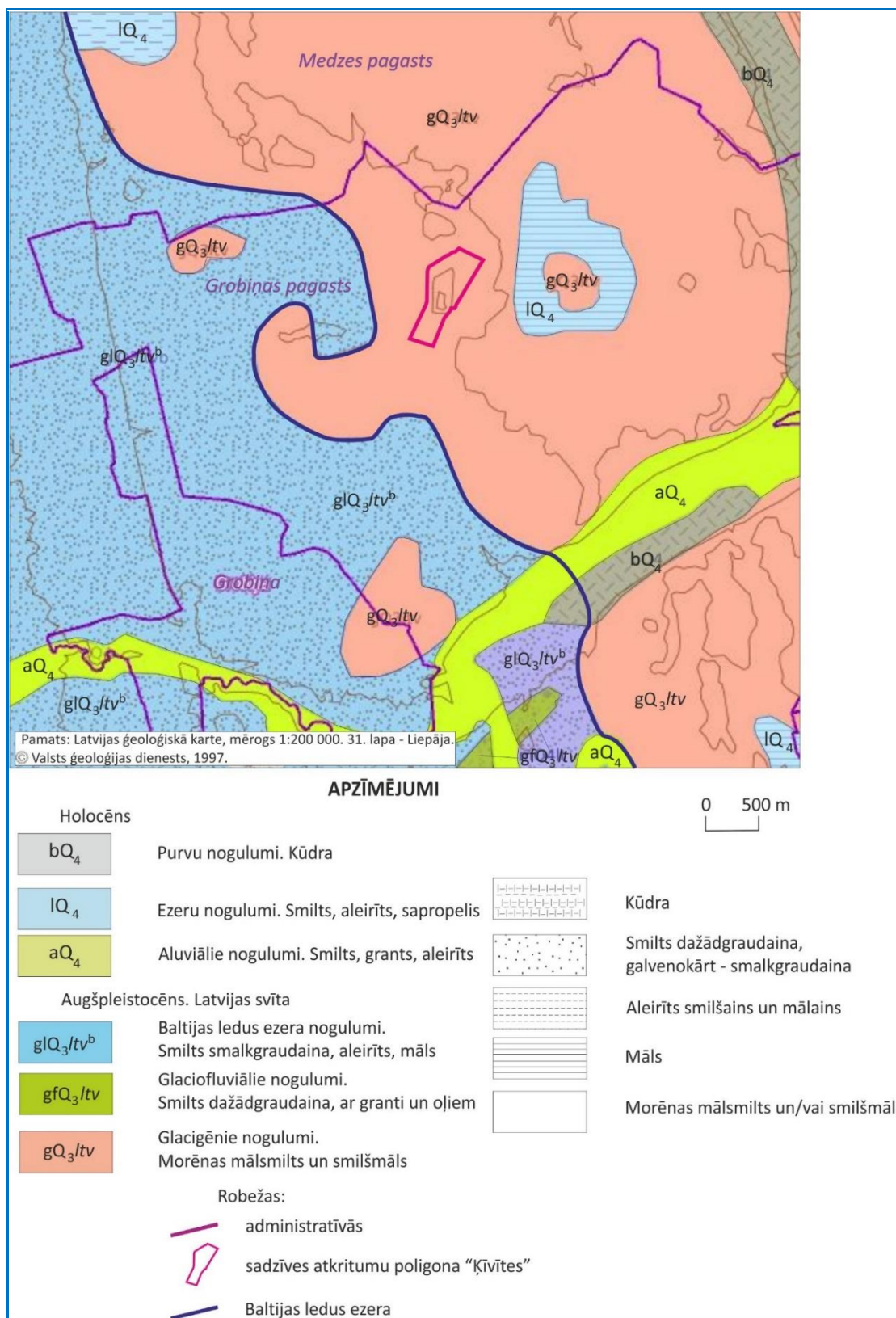
2.5. attēls. Kvartāra ģeoloģiskās kartes fragments
