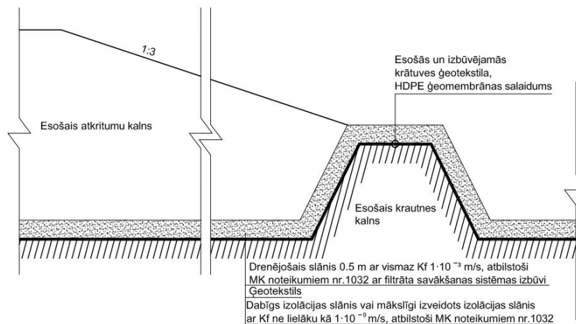
Griezums 3-3
