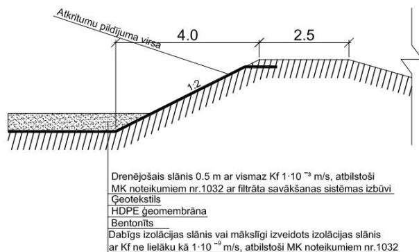
Griezums 2-2
