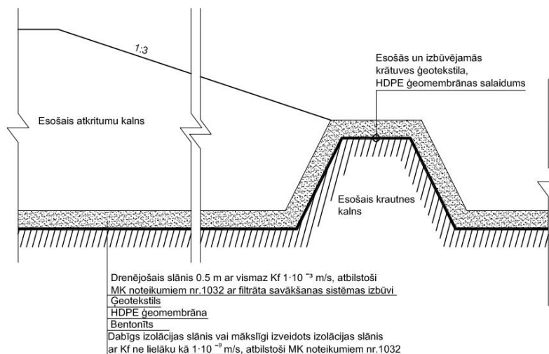
Griezums 3-3
