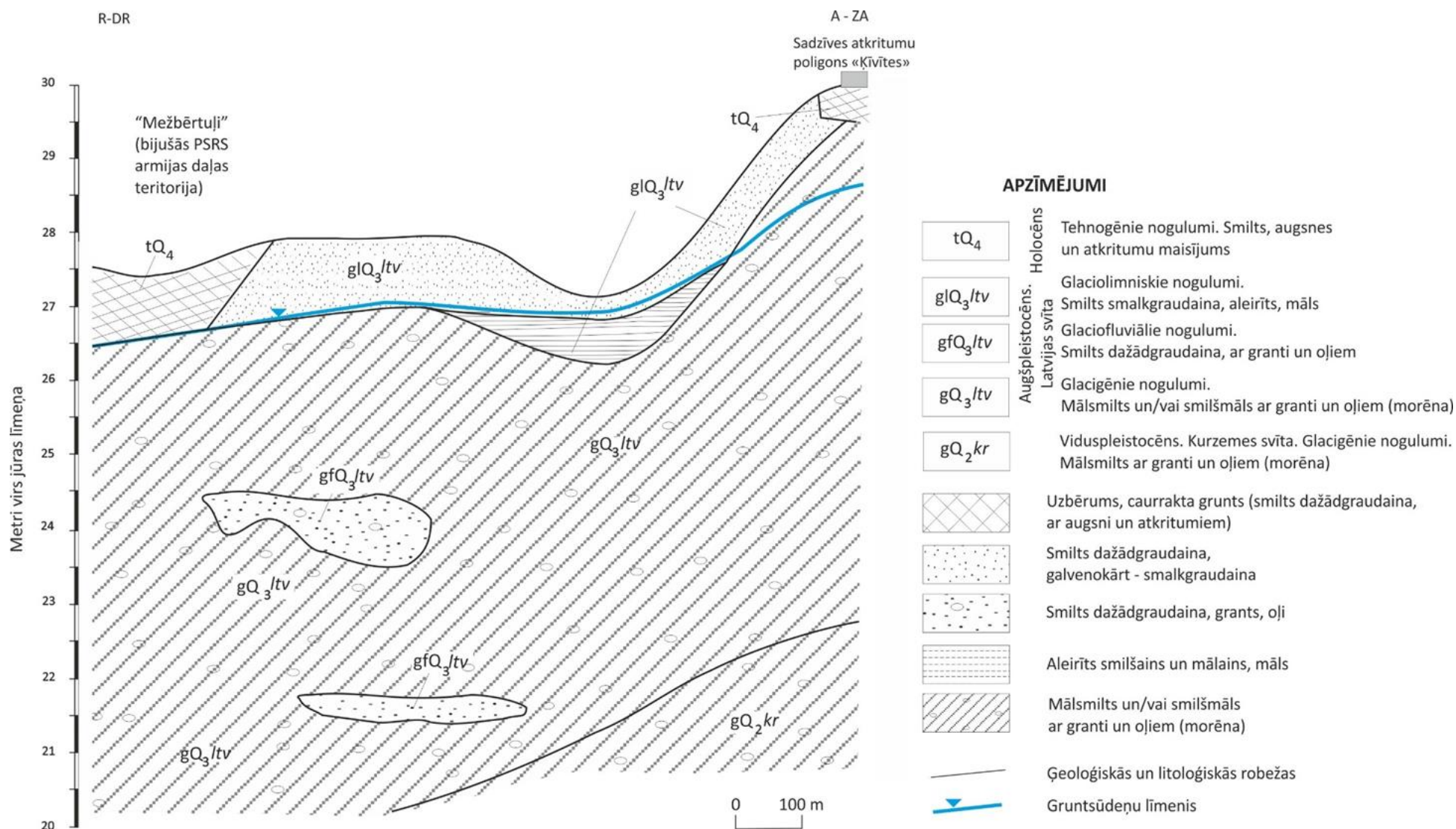
2.6. attēls. Kvartāra ģeoloģiskā griezumā augšdaļas principiālā shēma
