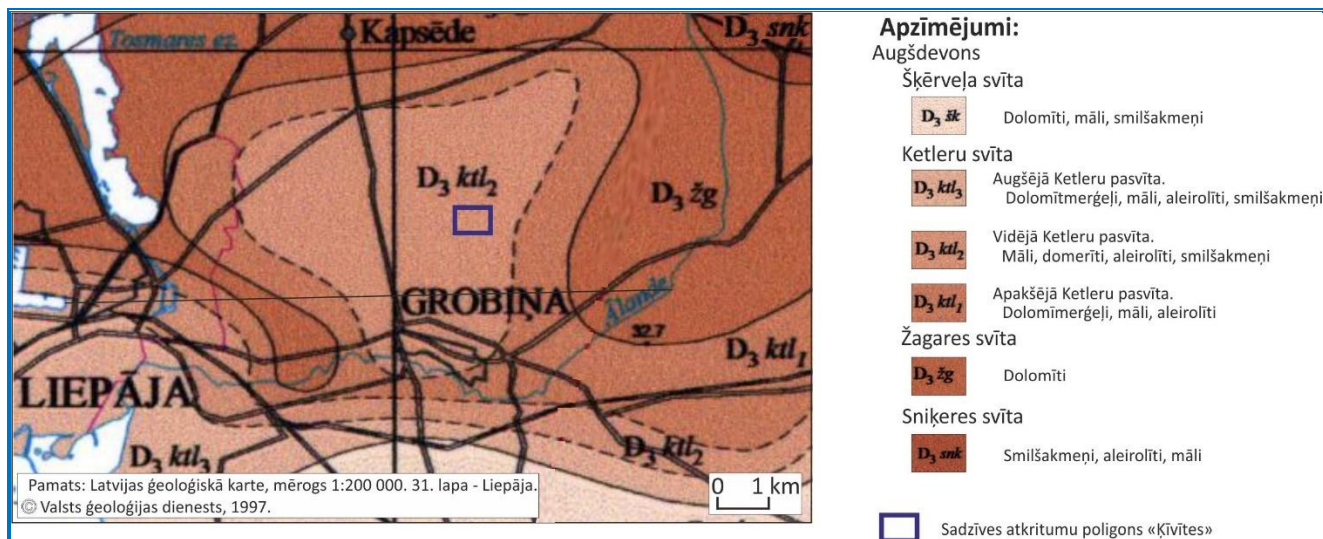
2.4. attēls. Pamatiežu ģeoloģiskās kartes fragments
