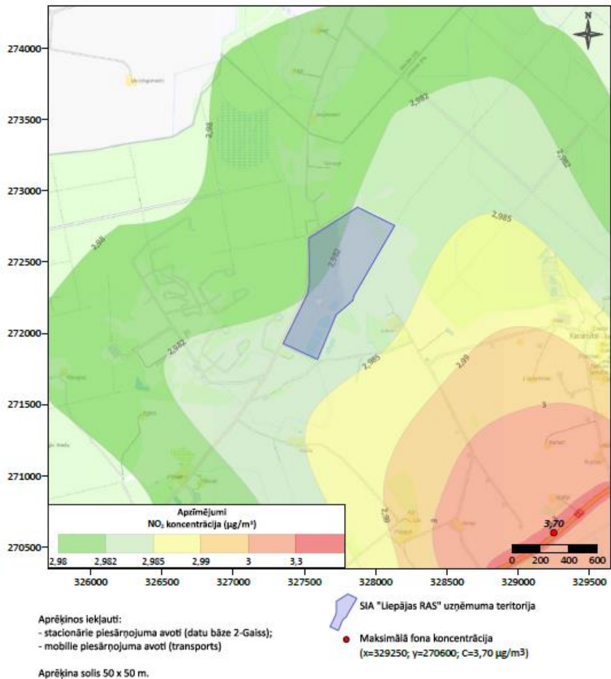
3.12. attēls. Slāpekļa dioksīda gada vidējo koncentrāciju novērtējums, fona piesārņojuma koncentrācija (avots: SIA "Ekosoft")
