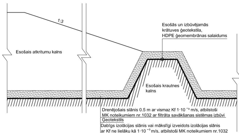
Griezums 3-3
