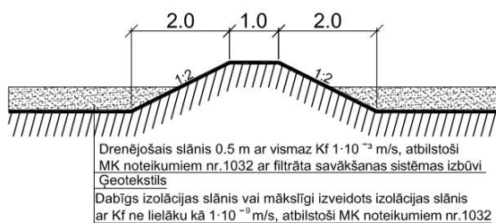
Griezums 2-2
